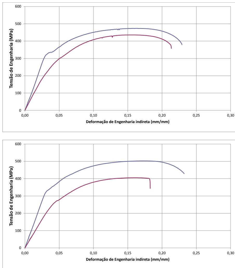
Figura 10. Gráficos tensão × deformação em CPs de tubos soldados antes e após ensaios os de corrosão acelerada: com consumível ER 70S-3 (esquerda); com consumível ER 80S-Ni3 (direita).
