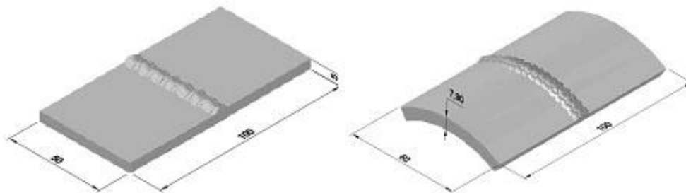
Figura 2. Dimensões do Corpos de prova após o corte oriundo: esquerda chapa; direita tubo.
