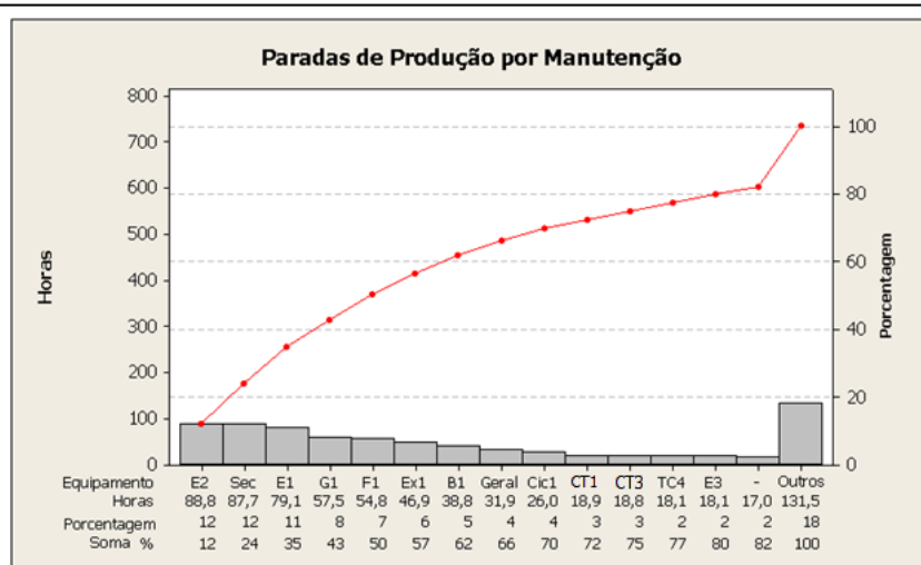
Figura 6. Paradas de produção para manutenção na planta industrial avaliada para implantação de uma correia transportadora tubular ( Pipe Conveyor ).
