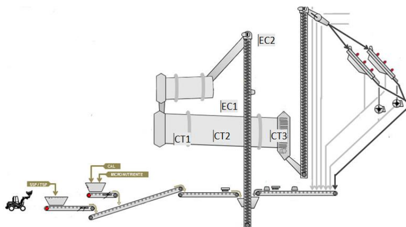
Figura 5. Fluxograma do processo avaliado para substituição por um sistema de correia tubular ( Pipe Conveyor ).
