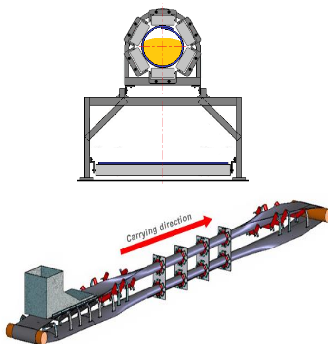
Figura 2. Roletes no padrão hexagonal formando a correia tubular ( Pipe Conveyor ) [8].
