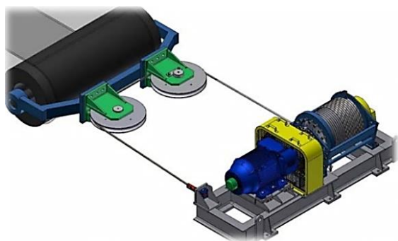
Figura 7. Esticador de correia do tipo Take up winch [15].
