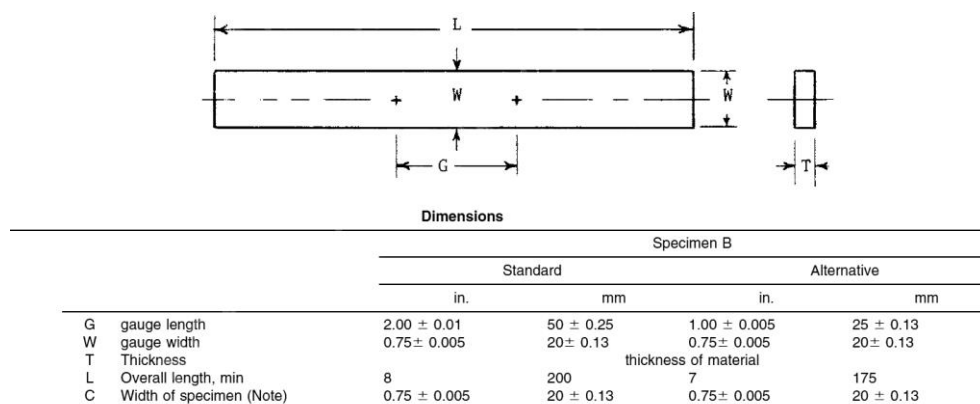
Figura 3. Dimensões dos Corpos de Prova empregados conforme ASTM E517 [5].
